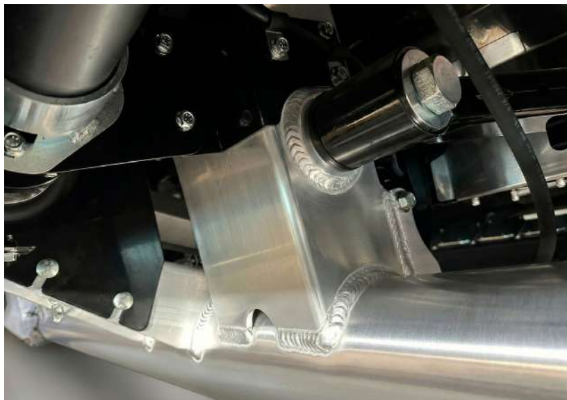
Châssis aluminium pour les modèles R XS.
