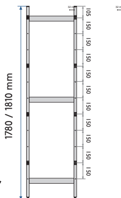
Échelle réglable sur 11 niveaux ou pas de 150 mm
