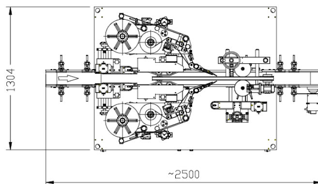
Etiqueteuse deux têtes
