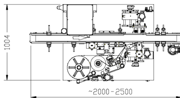
Etiqueteuse une tête
