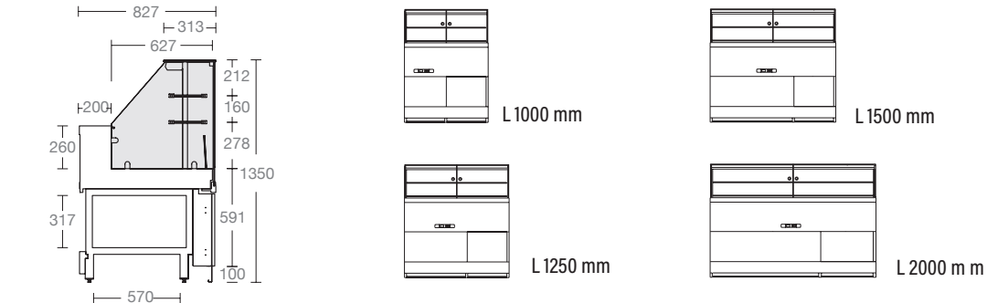
VETRINA REFRIGERATA STATICA CON MOTORE INCORPORATO H1350 D827 MM STATIC REFRIGERATED DISPLAY CASES WITH HERMETIC UNIT H1350 D827 MM
