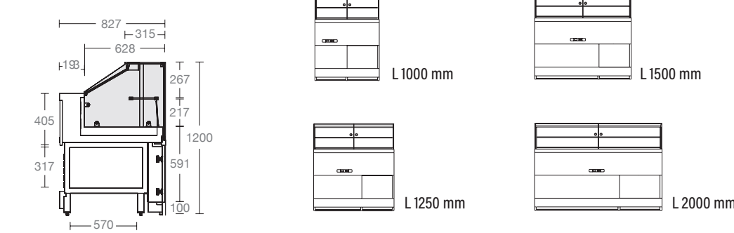
VETRINA REFRIGERATA STATICA CON MOTORE INCORPORATO H1200 P827 MM STATIC REFRIGERATED DISPLAY CASES WITH HERMETIC UNIT H1200 D827 MM
