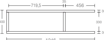
RETROALZATA BOTTIGLIERA "CESAR" P 236 "CICLOPE" BOTTLE COMPARTMENT D 236
