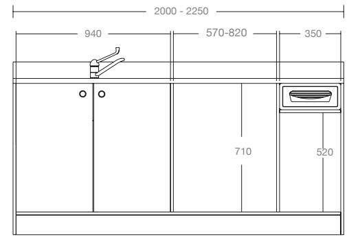
MODULO MACCHINA CAFFÈ RETRO COMBI CON 2 LAVELLI CAFFÈ MACHINE BACKCOUNTER COMBI WITH 2 SINK
