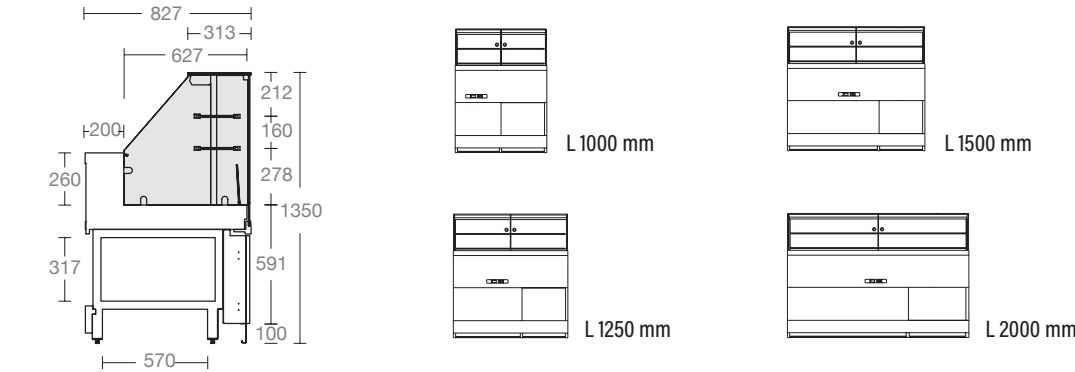
VETRINA REFRIGERATA VENTILATA CON MOTORE INCORPORATO H1350 P827 MM REFRIGERATED VENTILATED DISPLAY CASE WITH HERMETIC UNIT H1350 D827 MM
