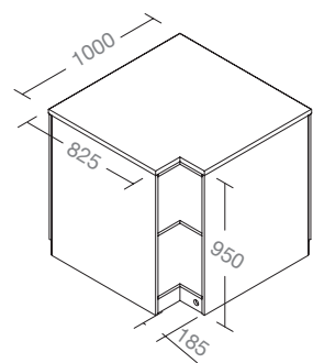
ANGOLO ESTERNO 90° L1000 H950 P1000 MM EXTERNAL CORNER 90° W1000 H950 D1000 MM
