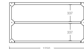
SCAFFALE PENSILE 1500 P 240 WALL SHELF 1500 D 240
