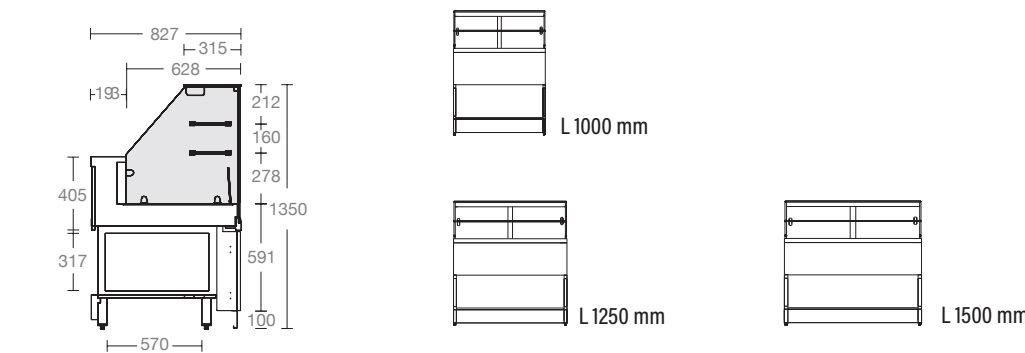
VETRINA CALDO SECCO H1350 P827 MM HOT DRY DISPLAY CASE H1350 D827 MM
