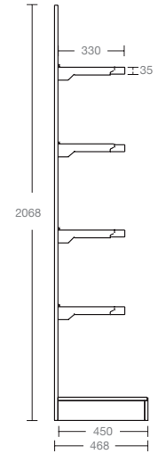
RETRO ESPOSITORE BACK DISPLAYER UNIT
