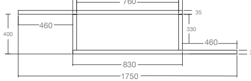
RETROALZATA BOTTIGLIERA ZETA P 236 ZETA BOTTLE COMPARTMENT D 236
