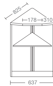
ANGOLO INTERNO 45° L795 H950 P825 MM INTERNAL CORNER 45° W795 H950 D825 MM
