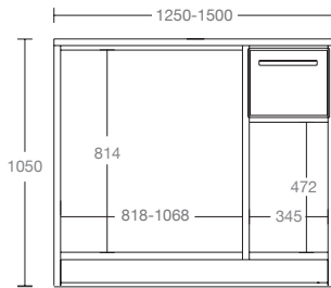
BASE PER MACCHINA CAFFÈ COFFEE MACHINE UNIT
