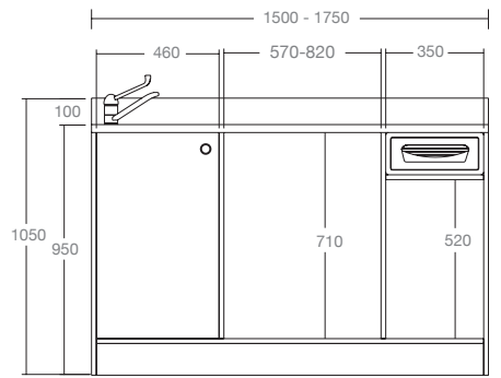
MODULO MACCHINA CAFFÈ RETRO COMBI CON 1 lavello CAFFÈ MACHINE BACKCOUNTER COMBI WITH 1 SINK
