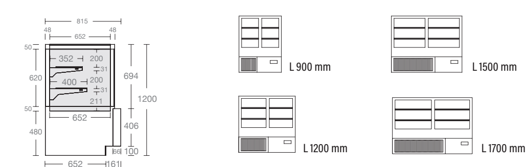
VETRINA REFRIGERATA VENTILATA CON MOTORE INCORPORATO H1350 P827 MM REFRIGERATED VENTILATED DISPLAY CASE WITH HERMETIC UNIT H1200 D827 MM
