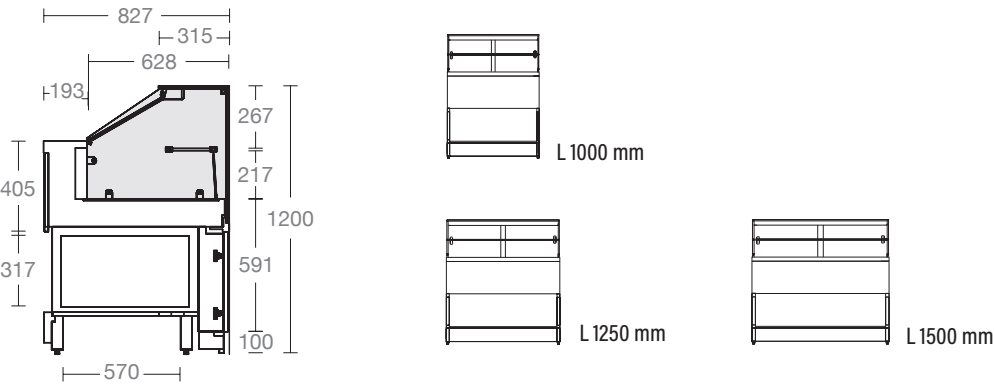
VETRINA CALDO SECCO H1200 P827 MM HOT DRY DISPLAY CASE H1200 D827 MM
