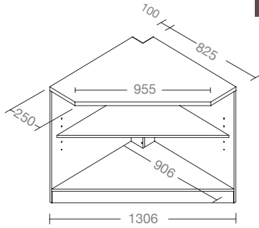
ANGOLO INTERNO 90° L925 H950 P925 MM INTERNAL CORNER 90° W925 H950 D925 MM
