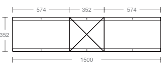
RETROALZATA BOTTIGLIERA "CROSS" P 200 "CROSS" BOTTLE COMPARTMENT D 200
