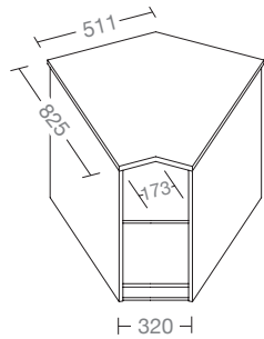
ANGOLO ESTERNO 45° L945 H950 P825 MM EXTERNAL CORNER 45° W945 H950 D825 Mmmm
