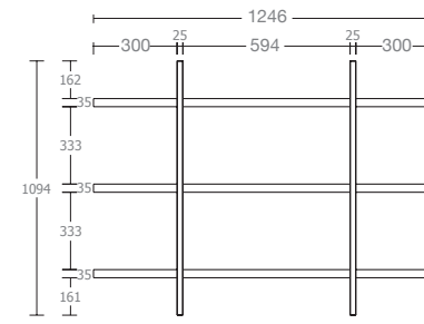
RETROALZATA BOTTIGLIERA "TRALIX" P 270 "TRALIX" BOTTLE COMPARTMENT D 270
