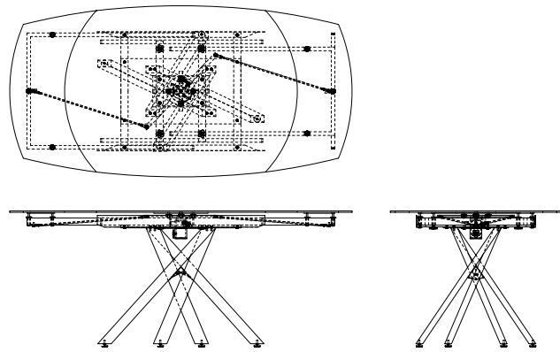
ÉTUDE DE LA TABLE DE REPAS KHEOPS
