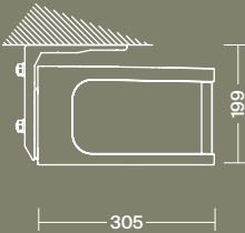
Ceiling installation Installation au plafond
