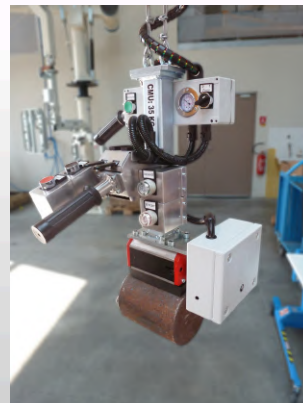
Pincettes de serrage ■ Palonnier à ventouses ■ Fourches ■ Plaque mousse aspirante ■ Mandrin pneumatique expansible ■ Aimant de levage
