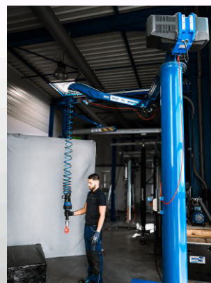
Équilibreur à poignée sensitive ■ Commande à vitesse progressive ■ Palan pneumatique à chaîne ■ Palan pneumatique à câble
