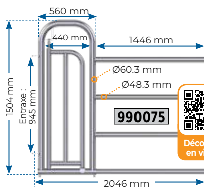
Avant passage homme L.V.4 avec portillon
