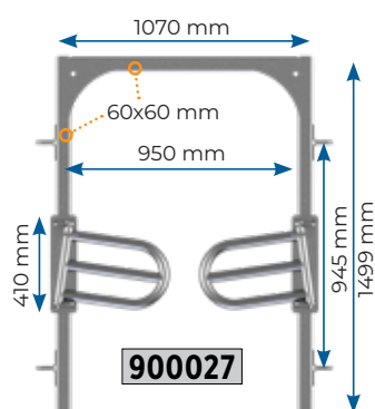
Panneau passage vache seul avec 2 portillons
