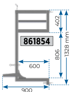
Protection abreuvoir bovin inox adaptable sur AR L.V.4-L.V.5
