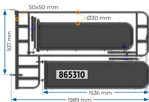
Panneau césarienne allaitement
