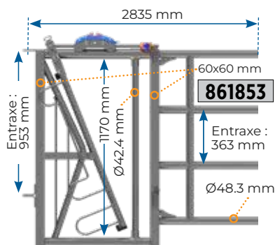
Avant cornadis insemination L.V.4 Elite
