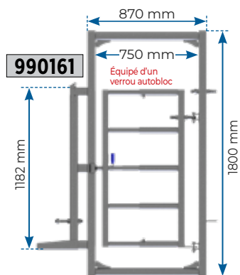
Passage homme secure
