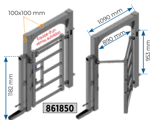
Passage évolutif pour veaux et bovins adultes
