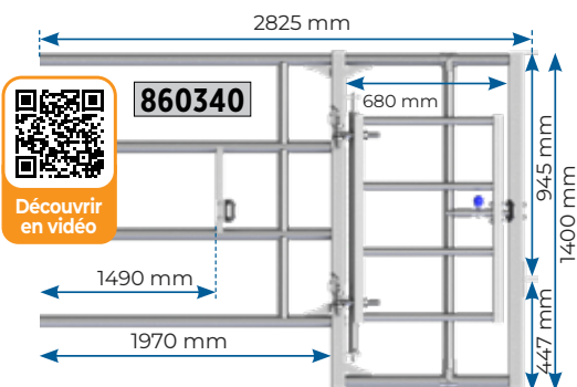
Avant passage sélectif à veaux L.V.4 avec portillon
