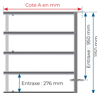
Arrière herbage standard
