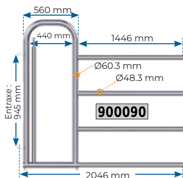
Avant passage homme L.V.4 sans portillon
