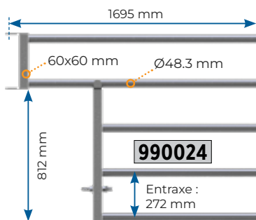
Avant découpe buse L.V.5 - 1m70
