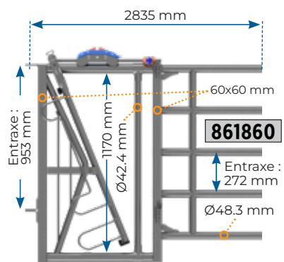
Avant cornadis insémination LV.5 Elite
