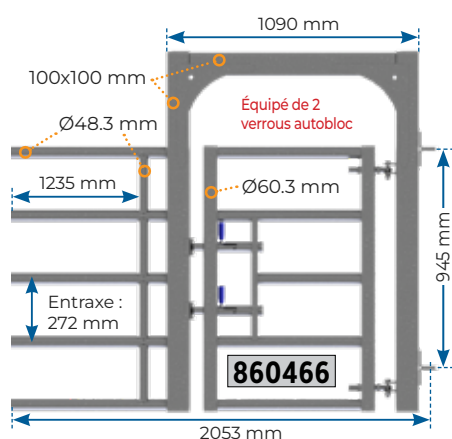
Avant passage gros bovins L.V.5
