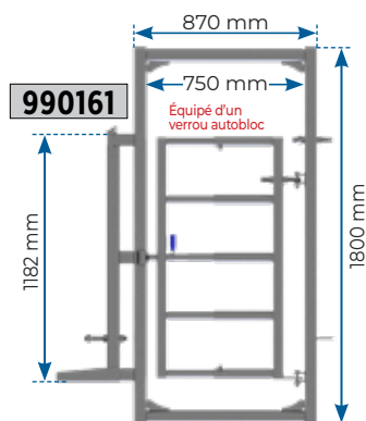
Passage homme secure
