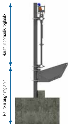
Exemple de montage avec une mangeoire en option
