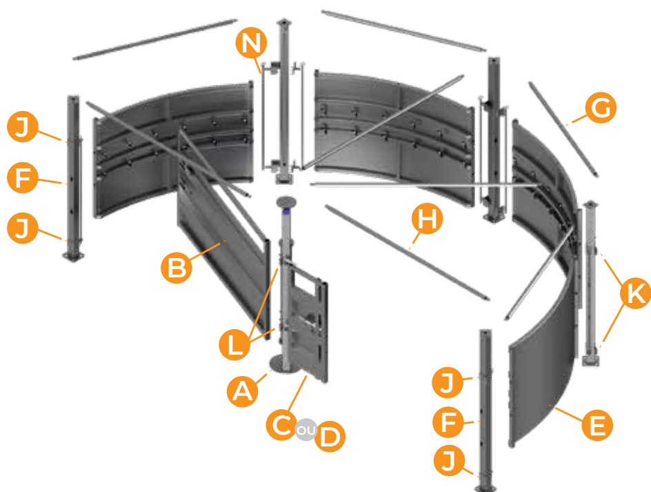
DÉTAIL 1/2 CIRCULAIRE ENTRÉE PAR CHICANE
