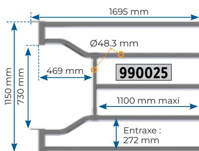
Avant découpe buvette L.V.5 - 1m70
