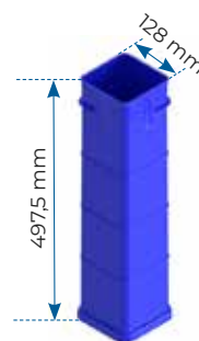
Réhausse de fourreau plastique 100X100
