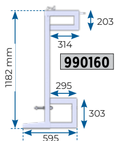
Protection abreuvoir adaptable tous modèles L.V.4-L.V.5
