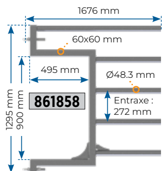
Avant L.V.5 découpe abreuvoir gamme inox
