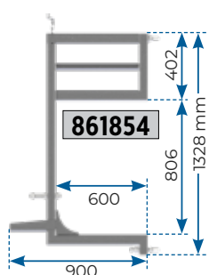
Protection abreuvoir bovin inox adaptable sur AR L.V.4-L.V.5
