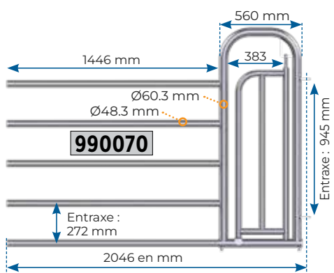
Avant passage homme L.V.5 avec portillon
