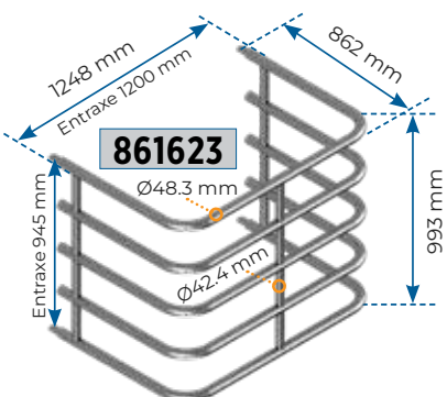
Protection abreuvoir L.V.5 VA
