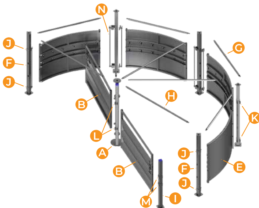
DÉTAIL 1/2 CIRCULAIRE ENTRÉE DIRECTE
