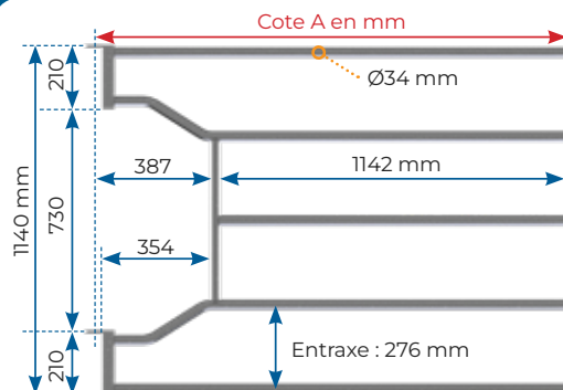
Avant découpe abreuvoir herbage
