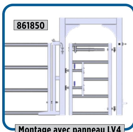
Montage avec panneau LV4
