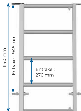
Portillon de service sans verrou
