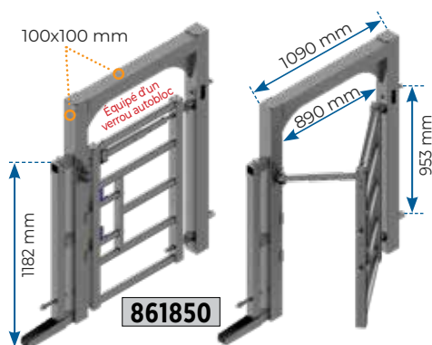
Passage évolutif pour veaux et bovins adultes
