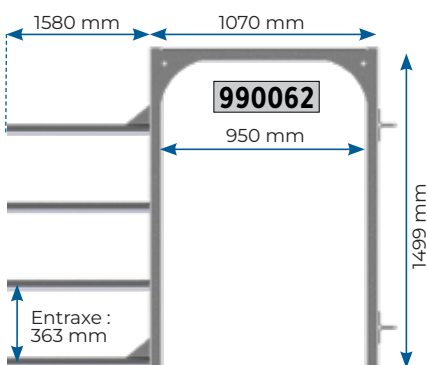
Avant passage vache L.V.4 réglable sans portillon
