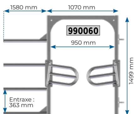
Avant passage vache L.V.4 avec 2 portillons
