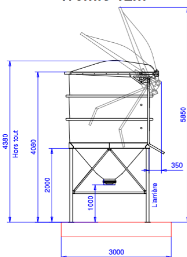
Trémie 12m 3
