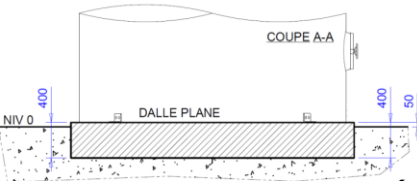
Plan de dalle pour cuve sur jupe porteuse :
