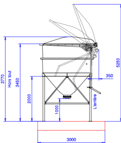
Trémie 9m 3
