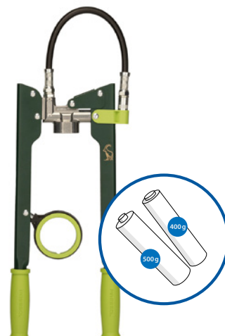
Pompe de graissage multi-cartouches 12 841 sans aimant, avec accessoires 12 841100 avec aimant et accessoires
