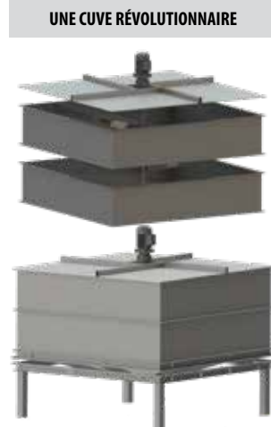
CUVE INOX DE MACHINE À SOUPE DE 2000L À 8000L UTILES
