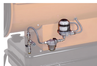
Kit raccordement réservoir extérieur
