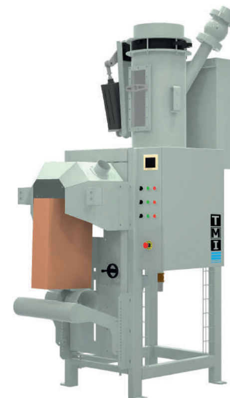
Ensacheuse manuelle par fluidisation pour sacs à valve, pour produits pulvérulents ou à faible granulométrie.
