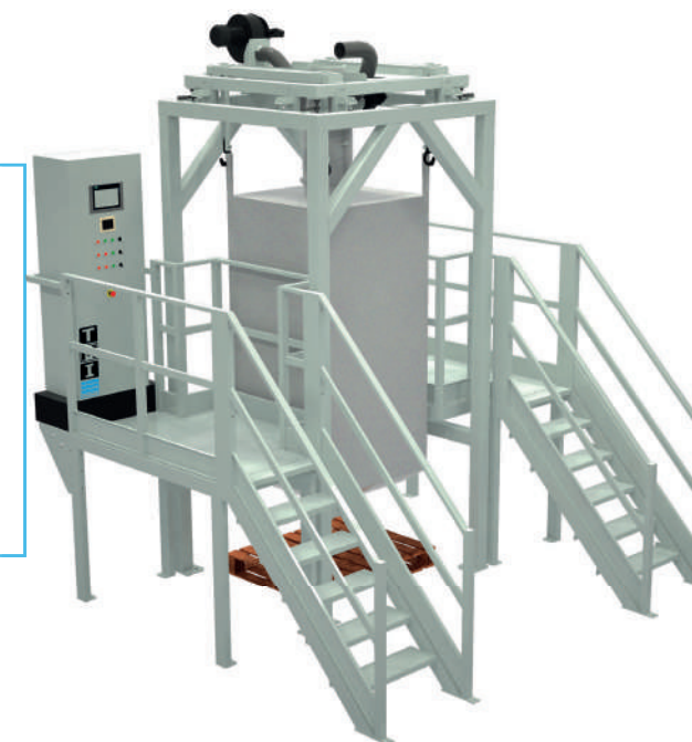
Poste de remplissage de big-bags simple.
