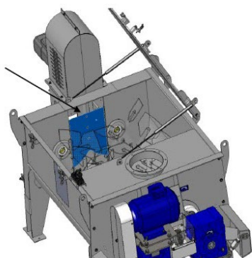
Trappe guillotine de régulation
