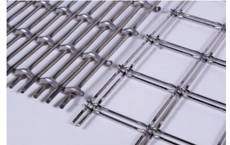
Grillages pré ondulés de tous types
