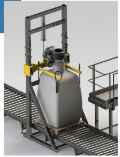
Remplisseuses Big Bag Big Bag Feeder
