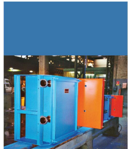
Sas à double clapets Double flap valves
