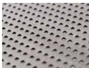
Tôle râpe pour lit fluidisé
